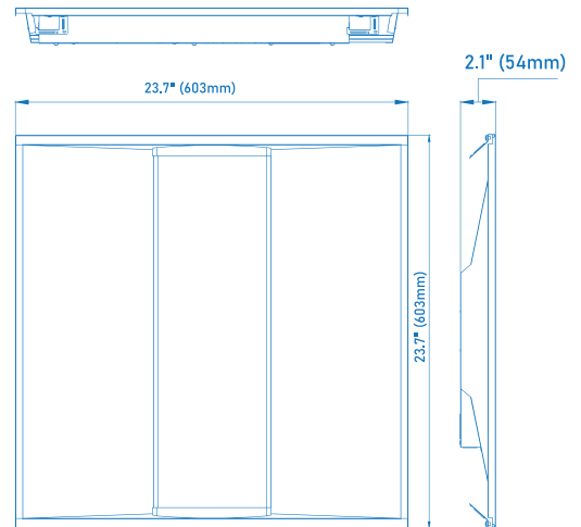
TDHE 22 LS42 - 2' x 2' Troffer
