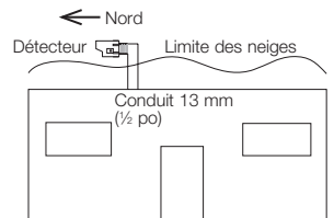
Montage du GRX-CESO
