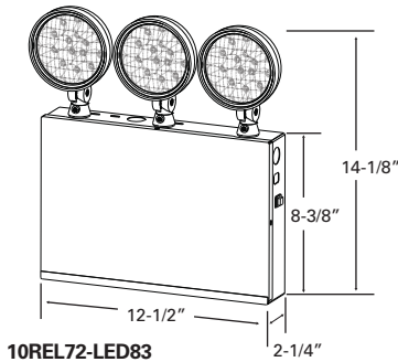
10REL72-LED83
